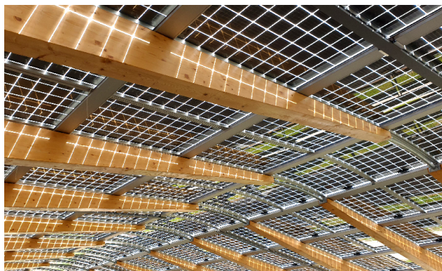
Abbildung 6: PV-Parkplatzüberdachung mit semitransparenten Glas-Glas-Modulen, die auch Tageslicht durchlassen.
